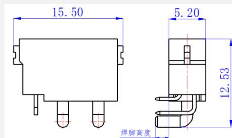
焊脚高度
