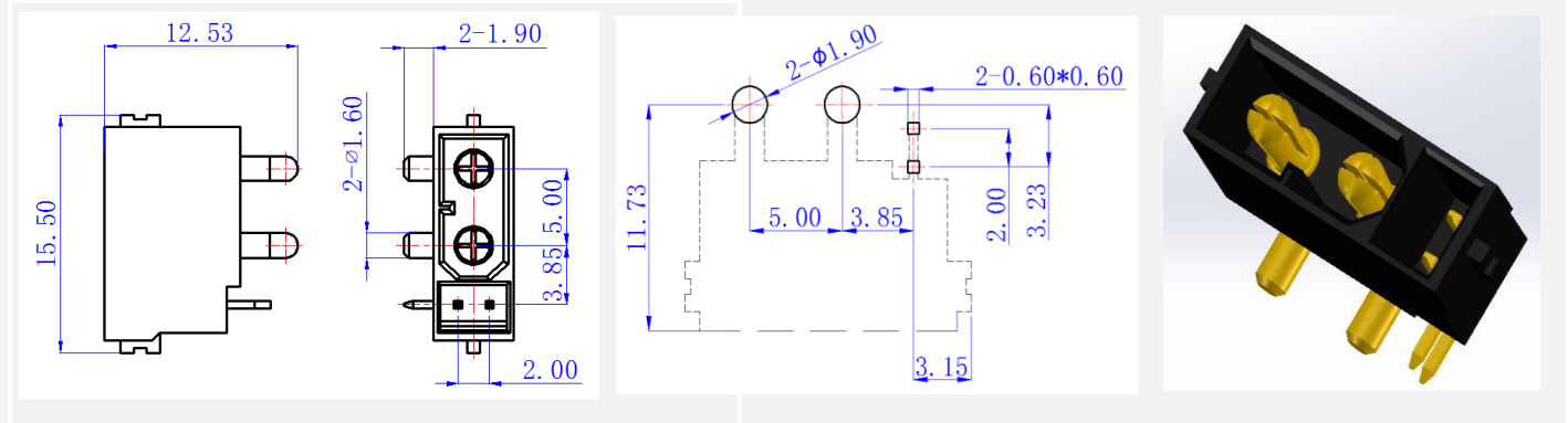
安装孔尺寸示意图
