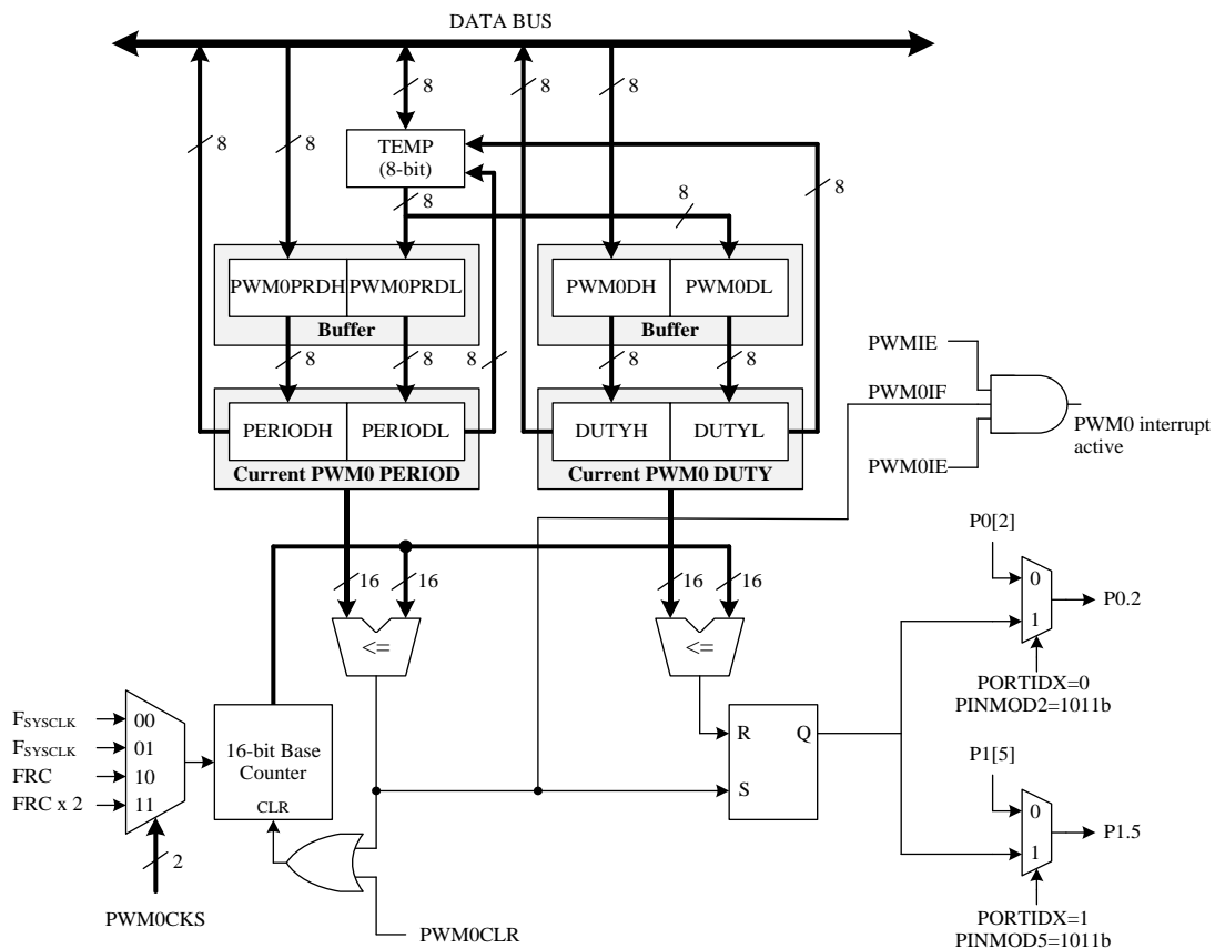
PWM0 结构
