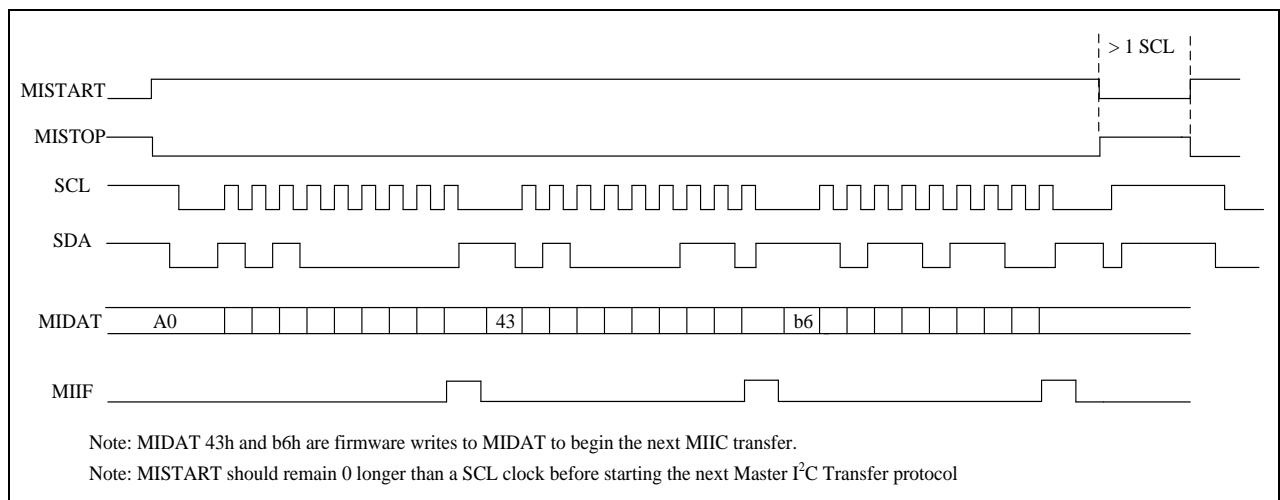
主发送时序
