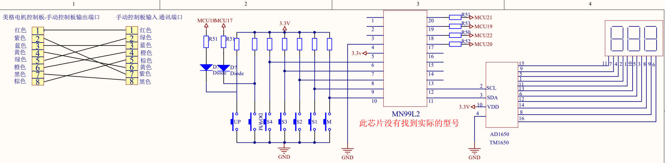
美格手动控制器与stm32F103C8T6T通讯电路图
