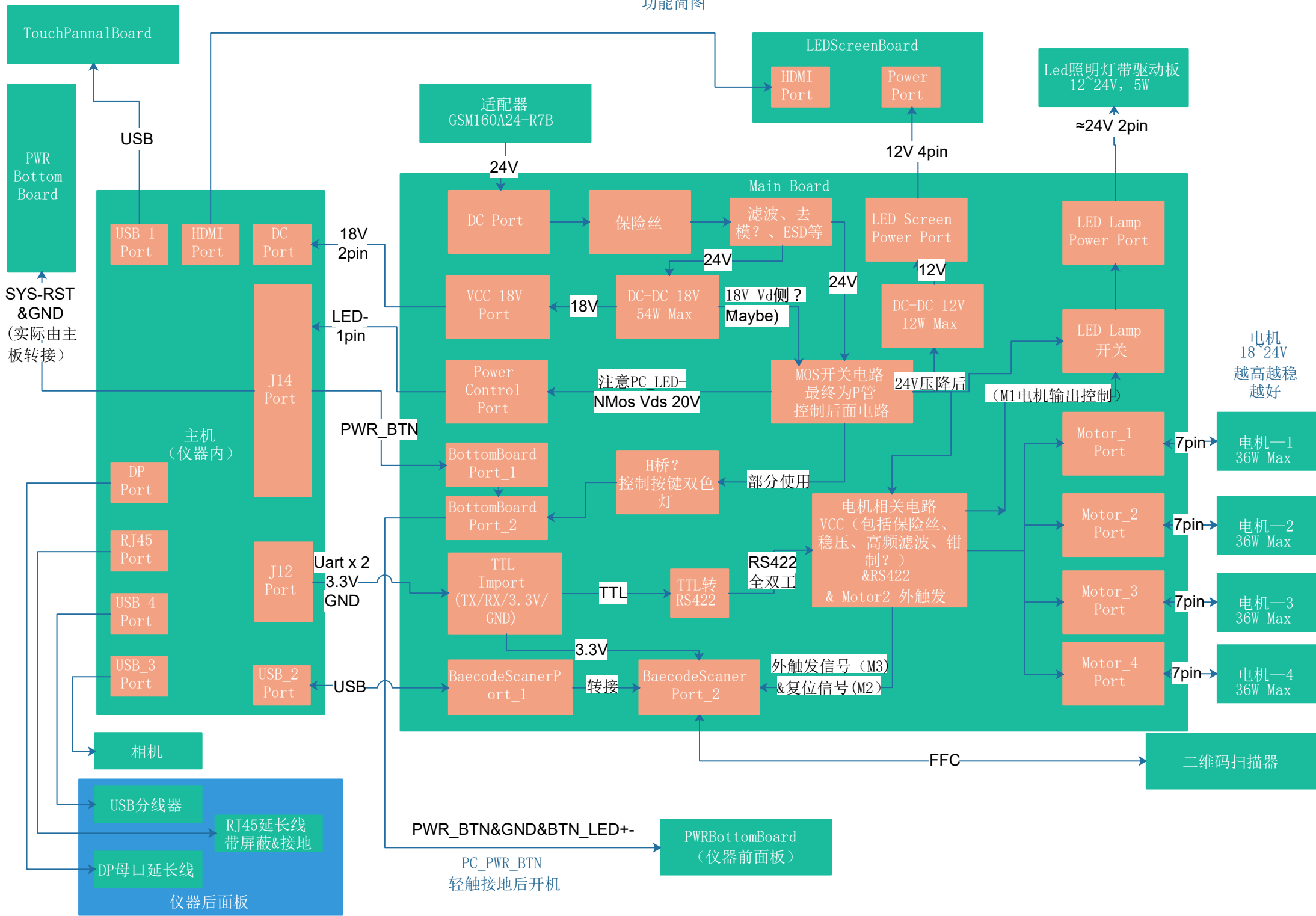
功能简图
