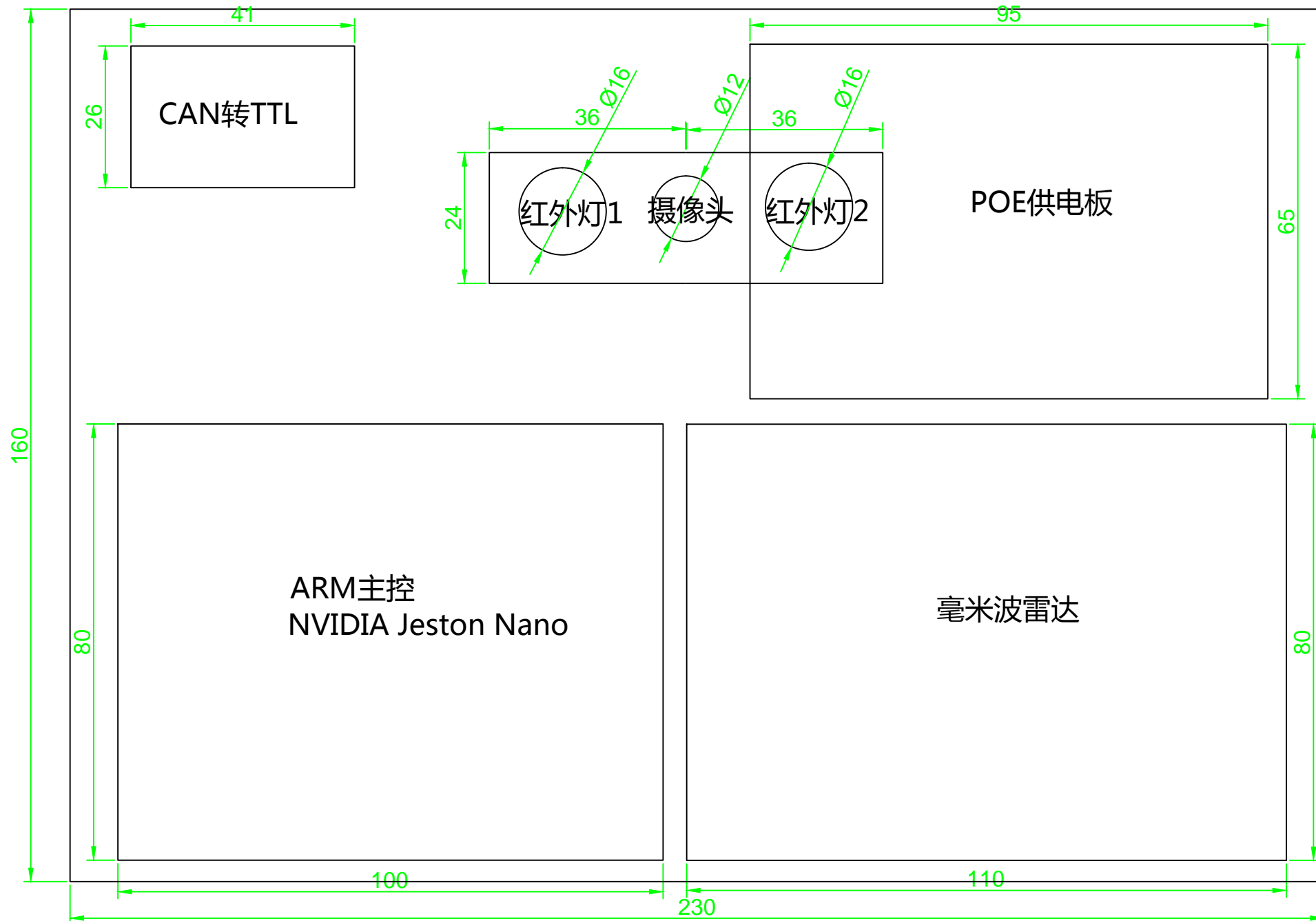
JOY SMART 可视雷达外壳布局平面示意图
