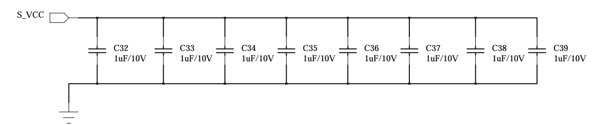
SDRAM_VCC FILWER
