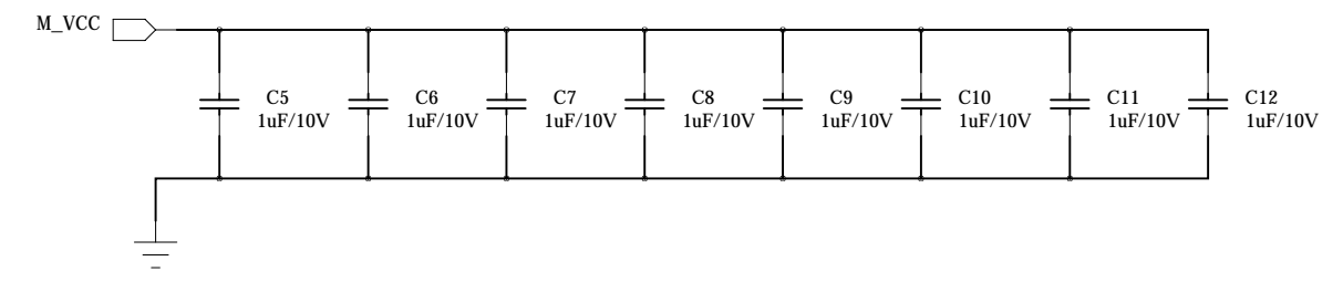
MCU_VCC FILWER
