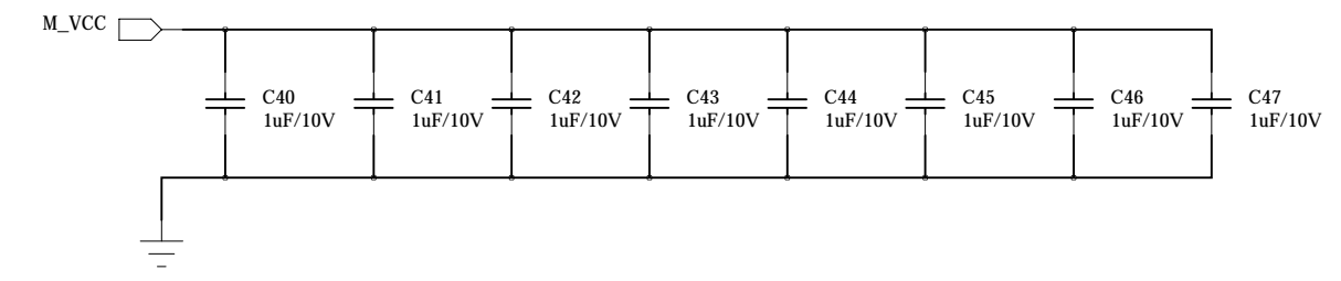
MCU_VCC FILWER
