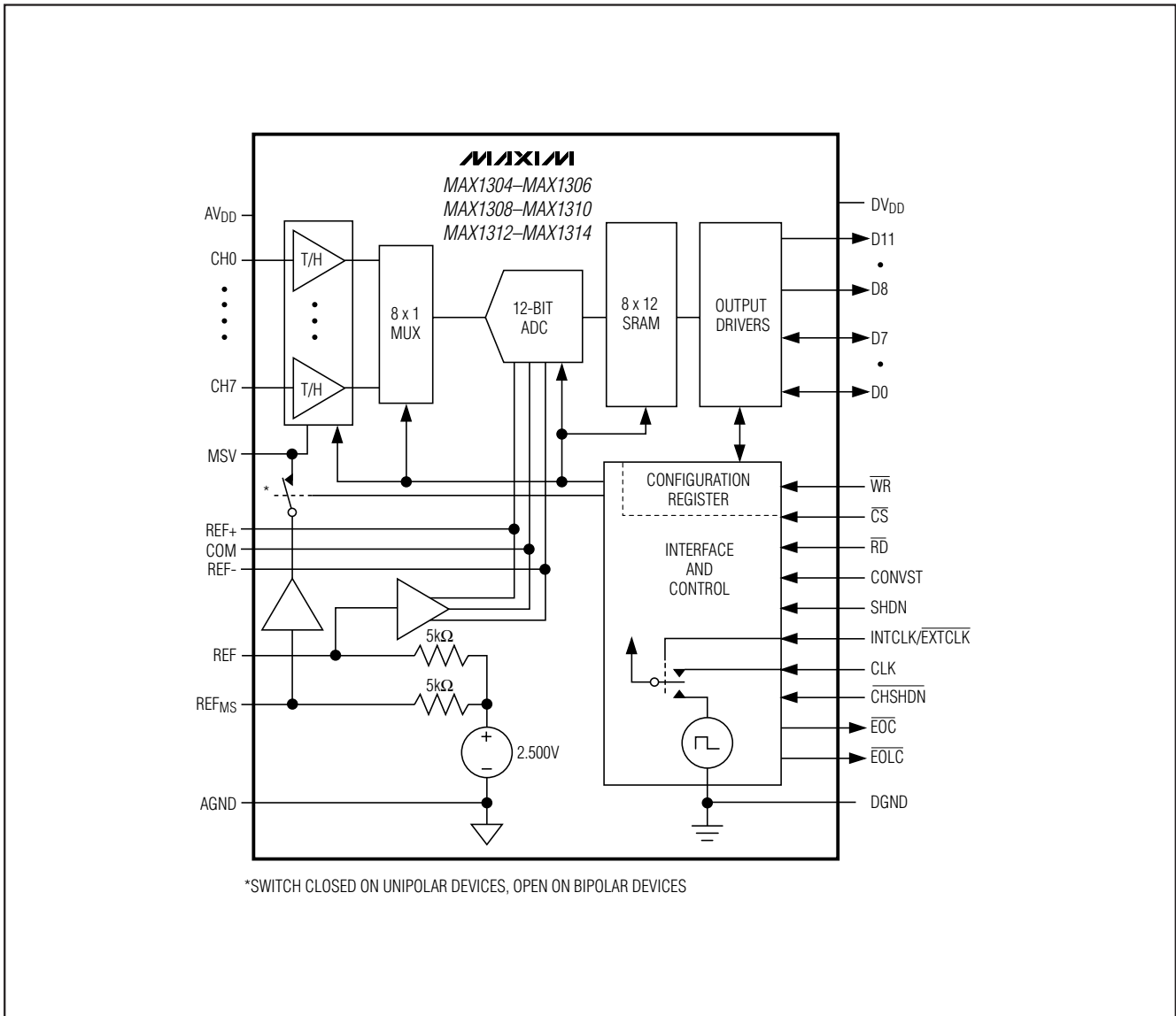
图2. 功能原理图
